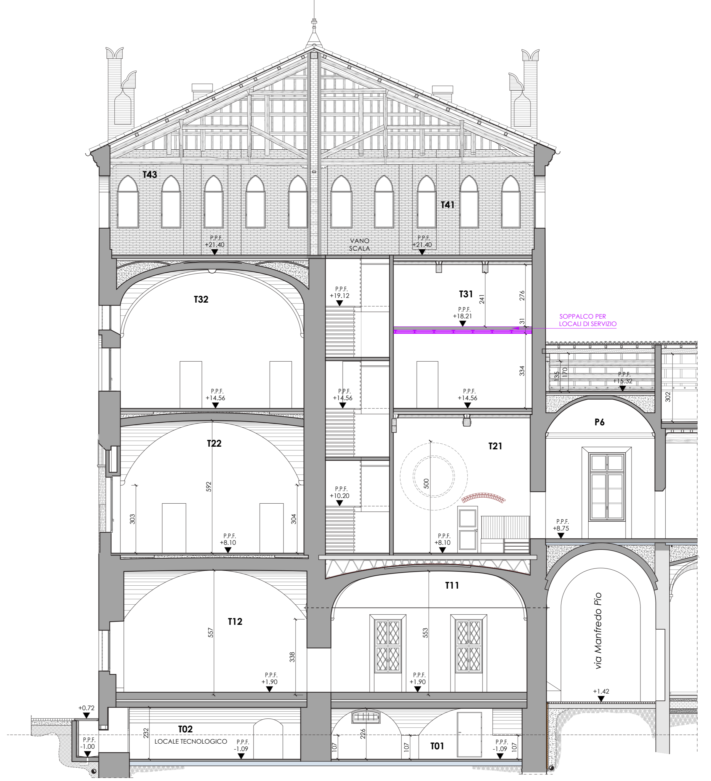
SEZIONE B-B'
