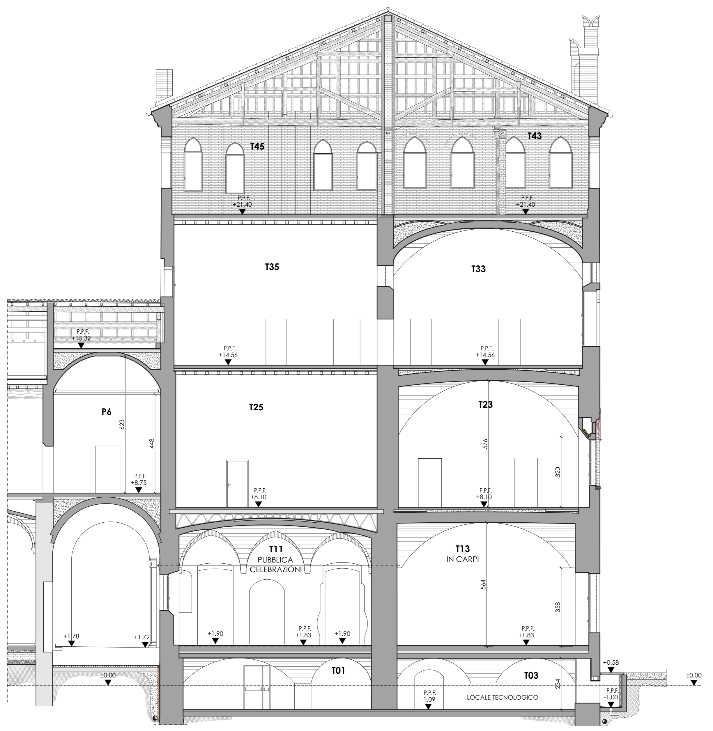
SEZIONE L-M'
