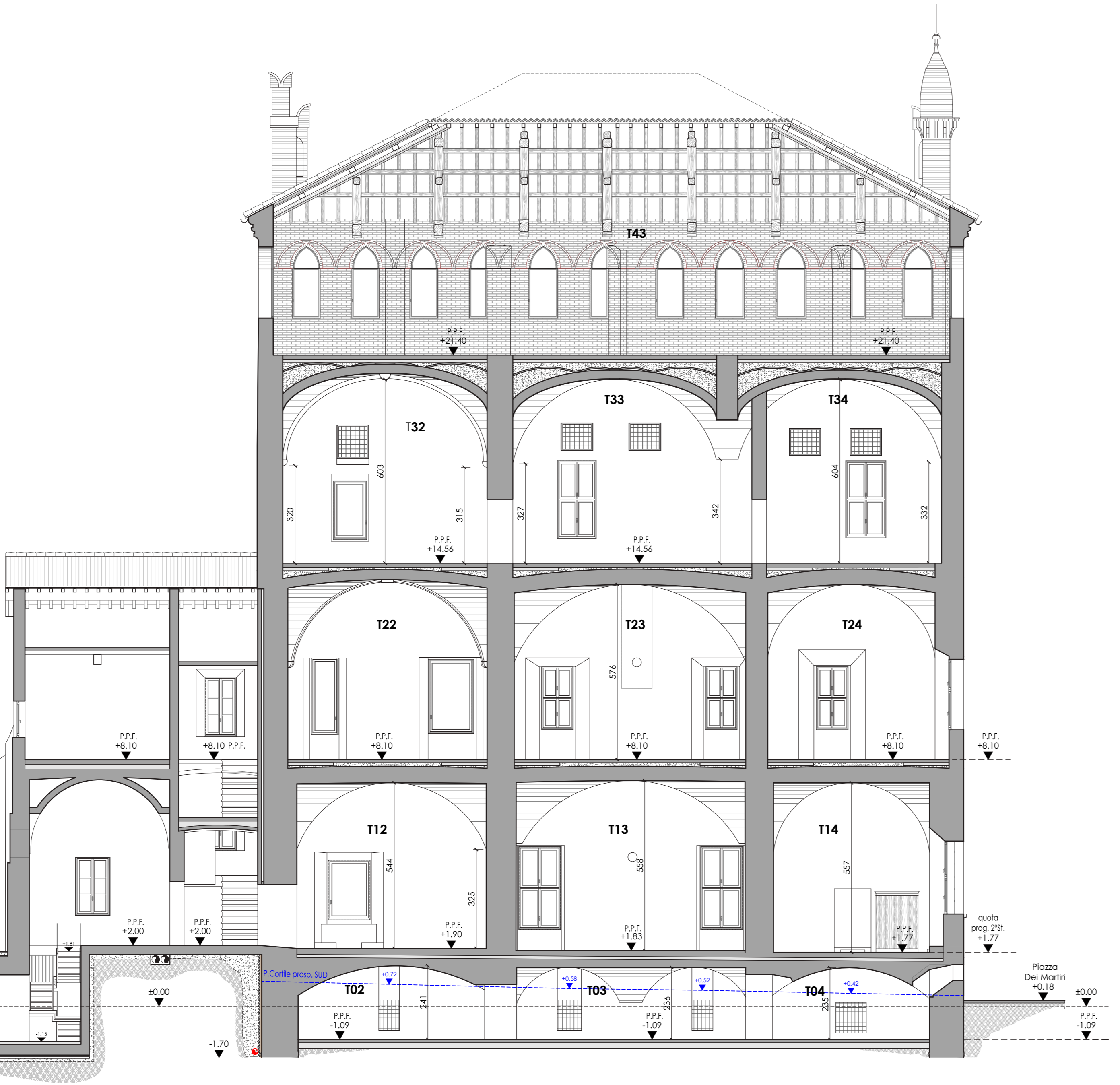
SEZIONE L-M'
