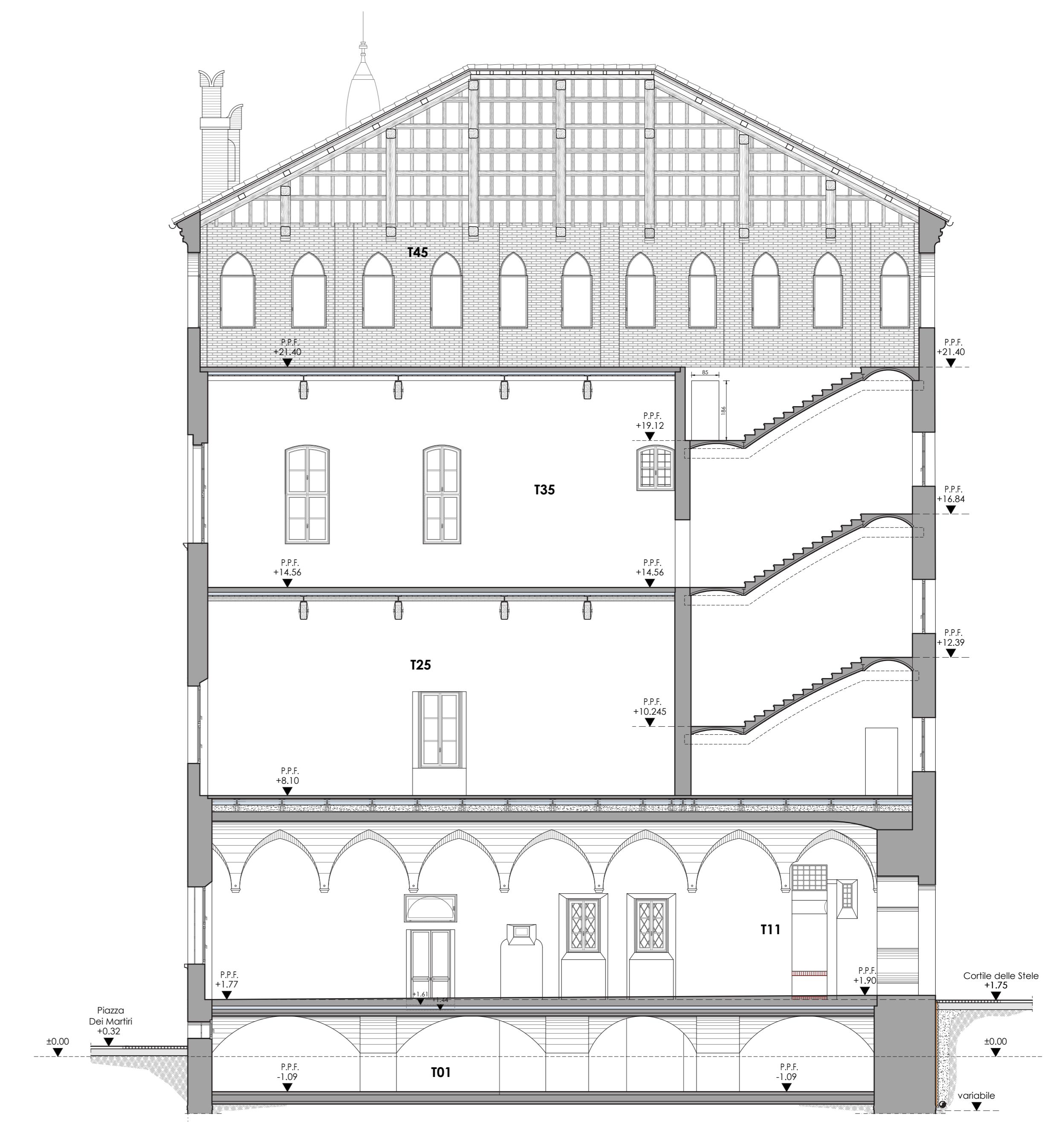
SEZIONE C-C'
