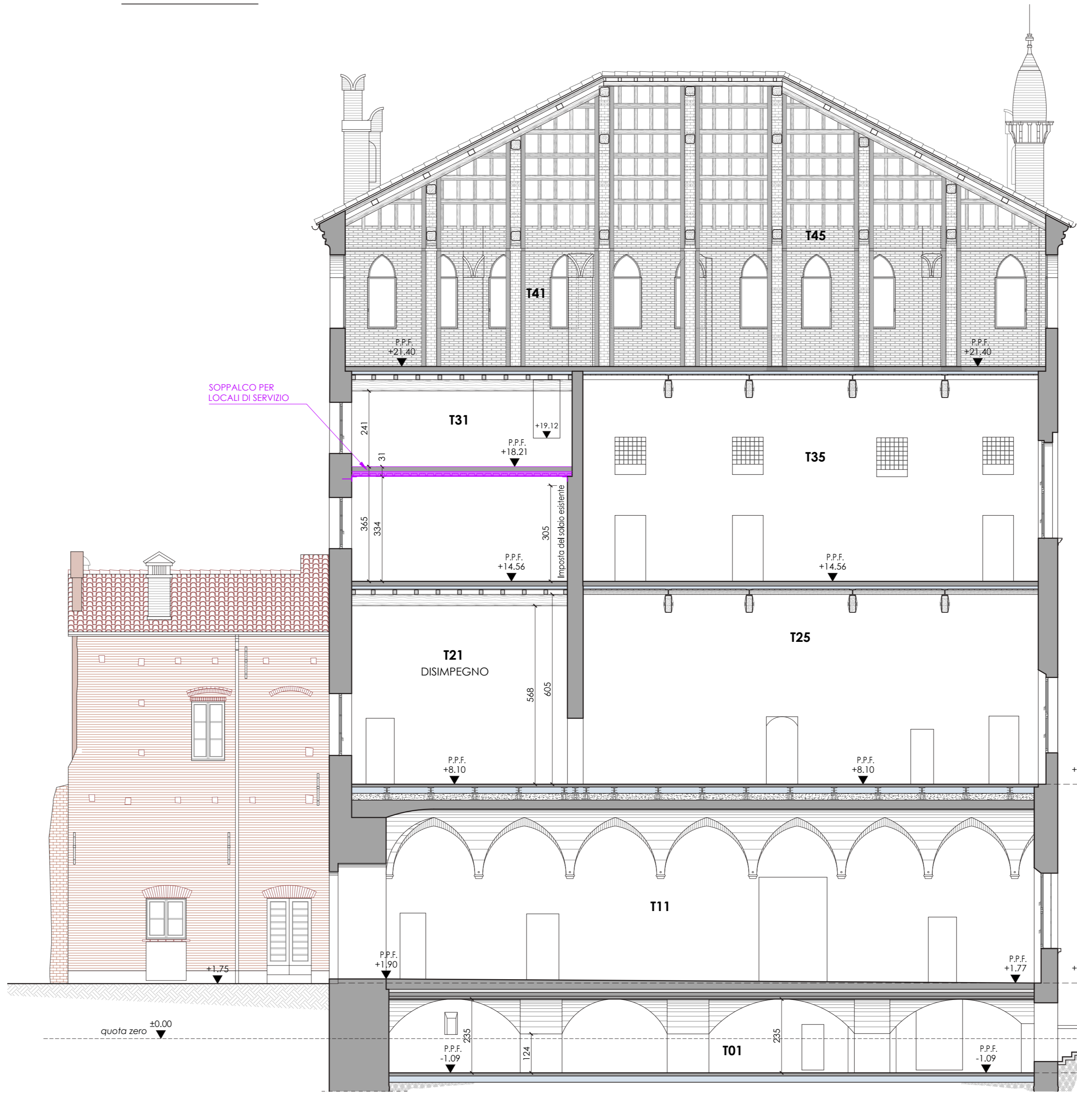
SEZIONE D-D'
