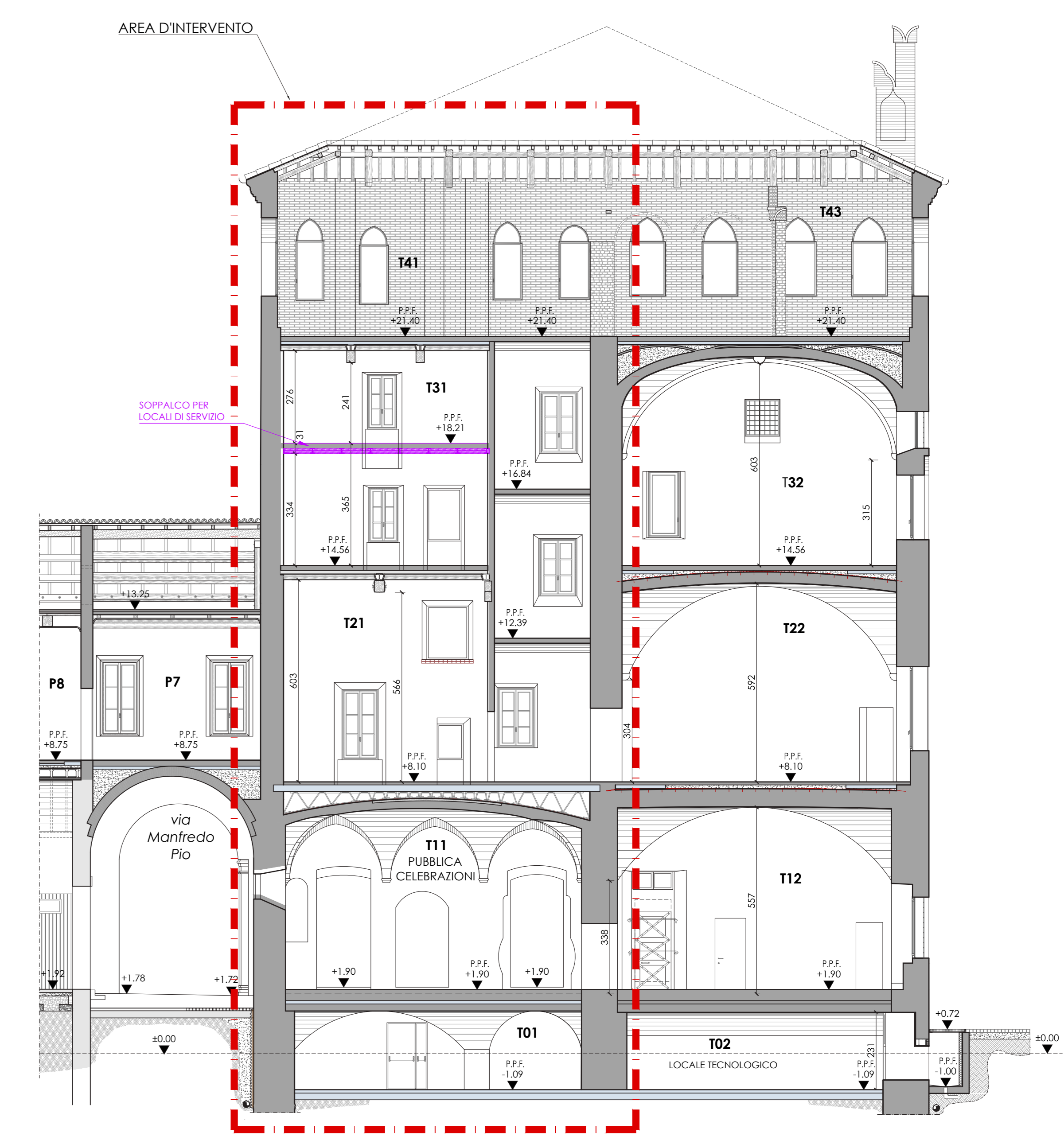
SEZIONE E-E'
